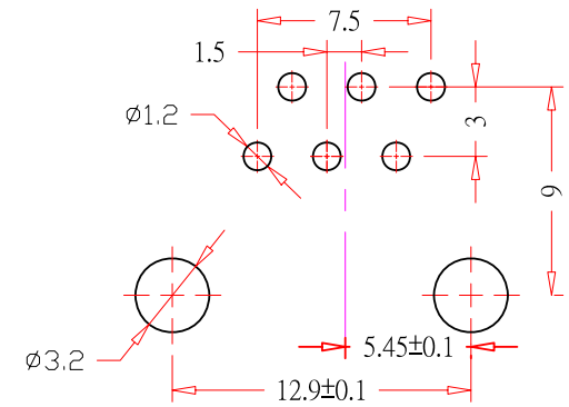
定位板孔位 PCB LAYOUT
