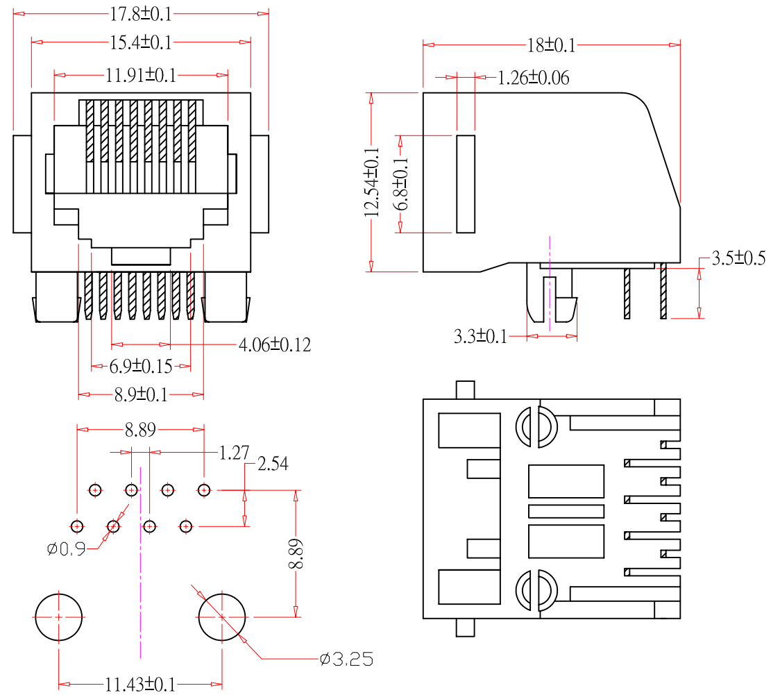
定位板孔位 PCB LAYOUT
