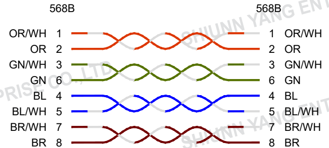
WIRING
