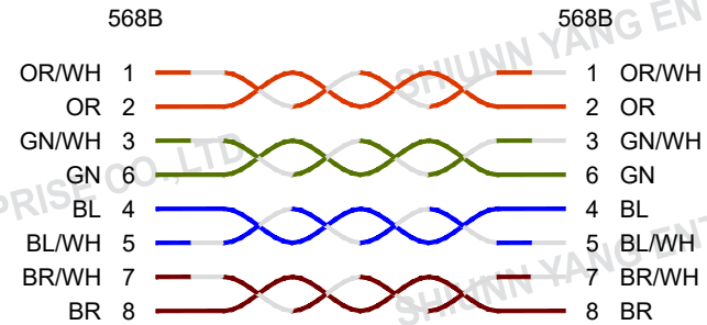
WIRING
