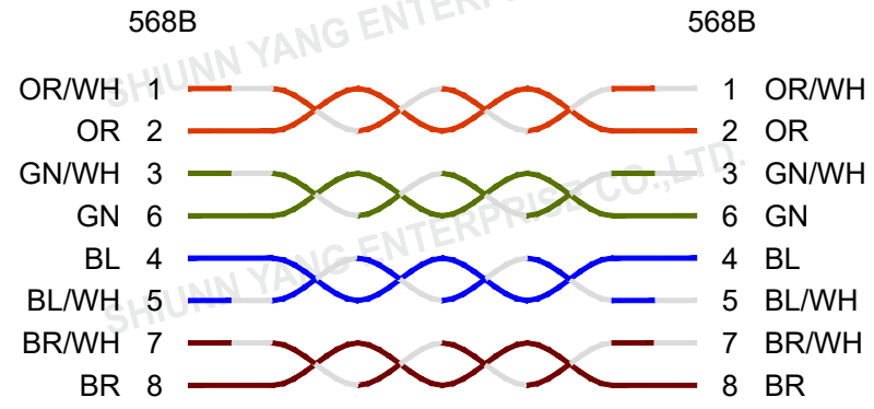
WIRING
