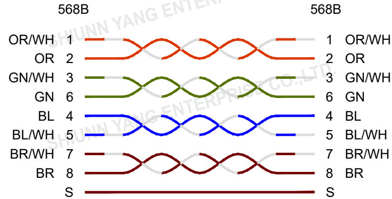
WIRING
