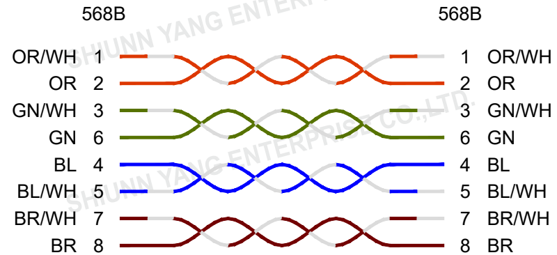
WIRING
