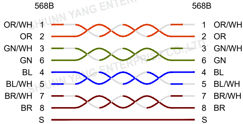
WIRING
