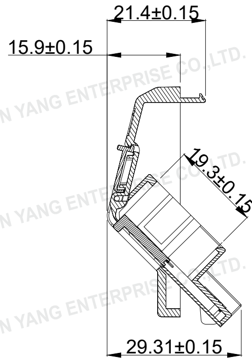
SCETION A-A
