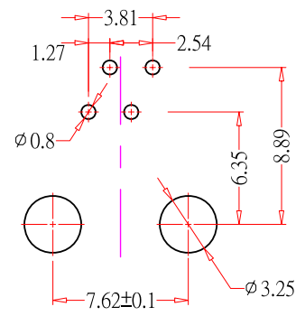
定位板孔位 PCB LAYOUT
